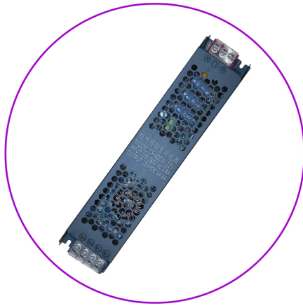
پاور سویچینگ اسلیم SI۱۰۳ خروجی ۱۲ ولت ۴۰۰ وات ۳۳ آمپر ۳۰۰ وات ۲۵ آمپر ۲۰۰ وات ۱۶/۷ آمپر ۱۰۰ وات ۸/۳ آمپر ۶۰ وات ۵ آمپر
